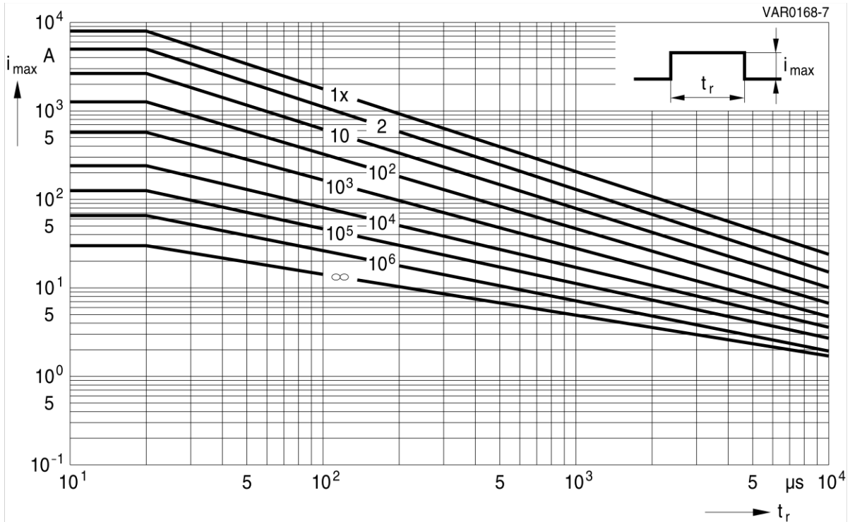
SIOV-S20K130 ... K320
