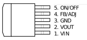
TO-263
